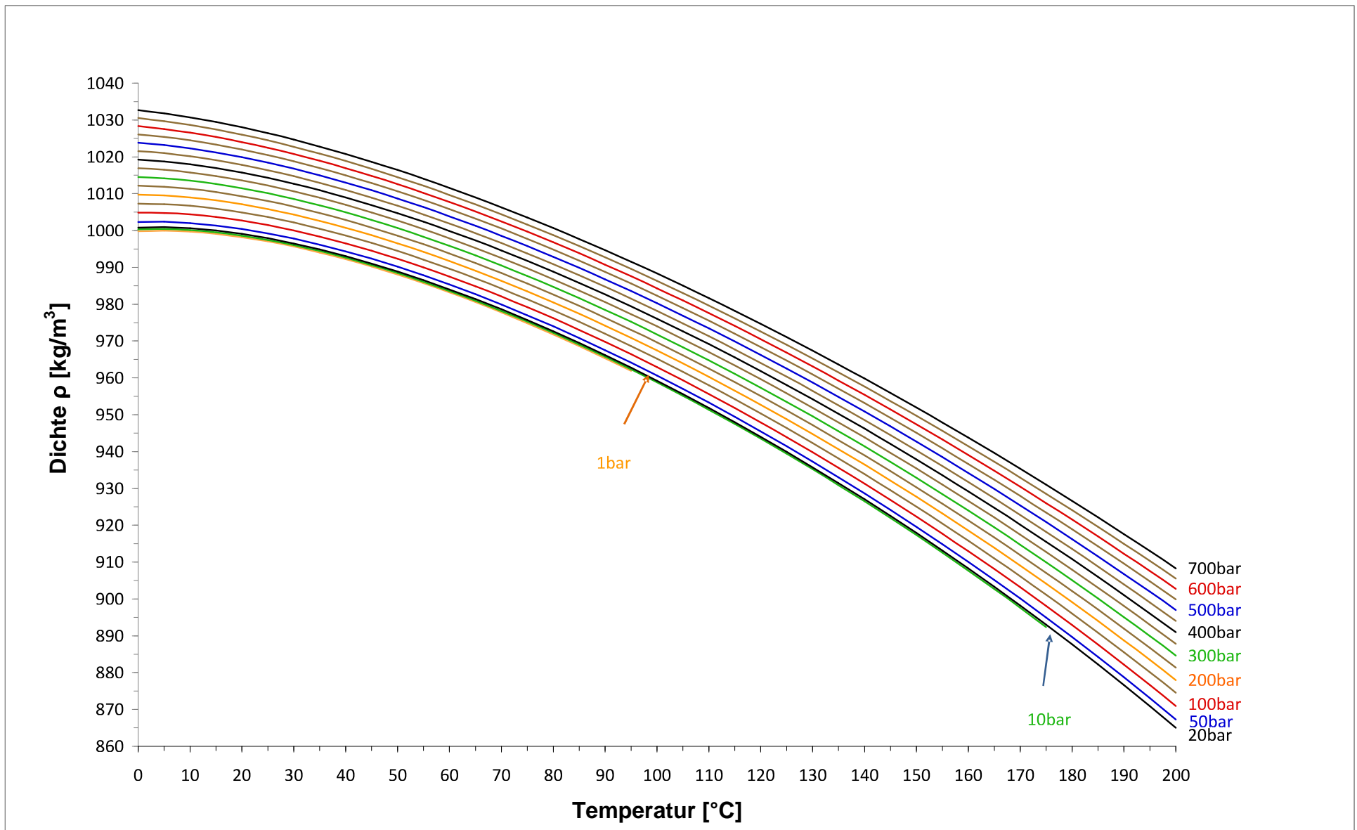
Abhängigkeit der Dichte reinen Wassers von Druck und Temperatur, nach Wagner & Kretschmar (2008)
